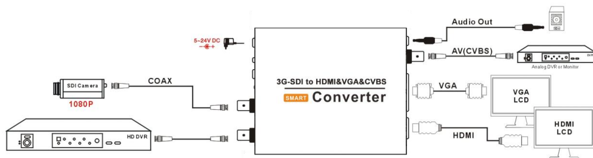
SD/HD/3G-SD-HDMI&VGA&AV 多功能转换器
