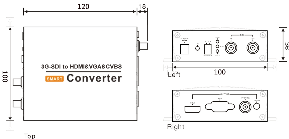
SD/HD/3G-SD-HDMI&VGA&AV 多功能转换器
