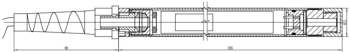
图 1 CHR. WYZ-1 型压力水位计外形图
