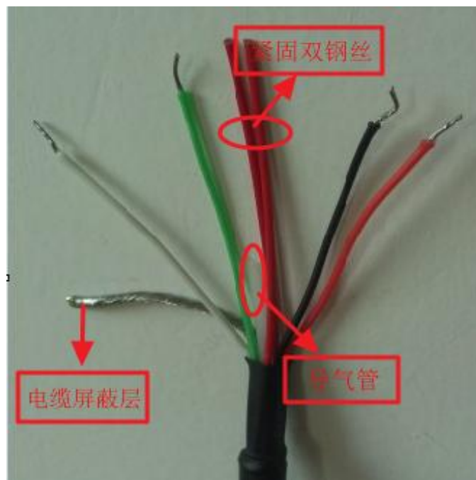
图 3 产品用户端电缆接口
