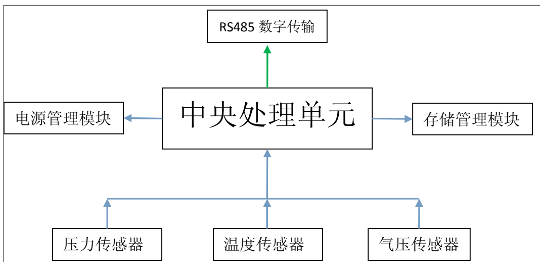
图 2 CHR. WYZ-1 型压力水位计原理框图
