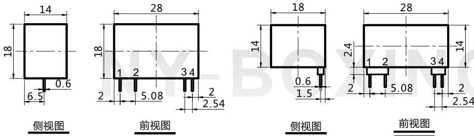
NEEx-Axx-1H(立式)
