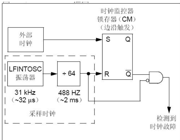
图 4-9：FSCM 框图
