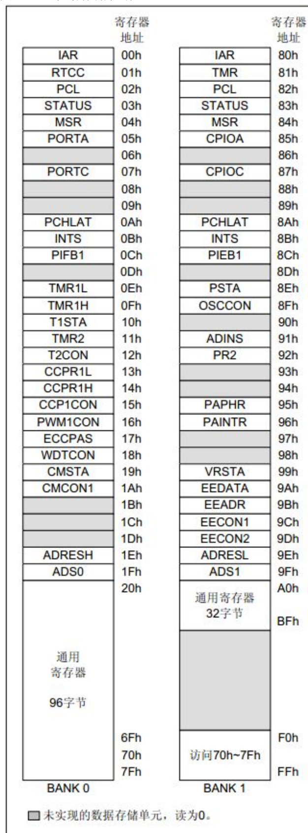
图 2-2: 数据存储映射
