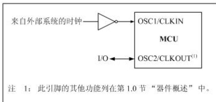
图 4-4-2: 外部时钟（EC）模式的工作原理
