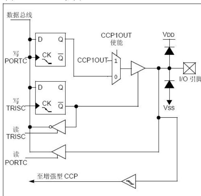
图 6-5-6: PC5 框图
