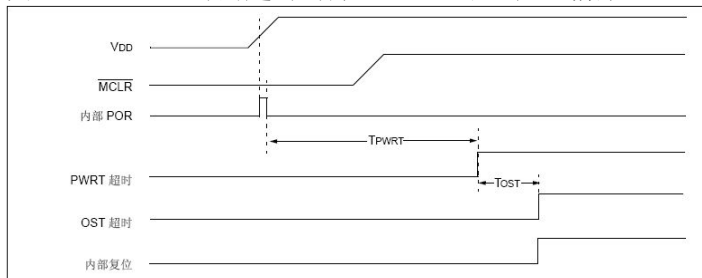
图 3-7-1: 上电时的超时时序 (MCLR 延时): 情形 1
