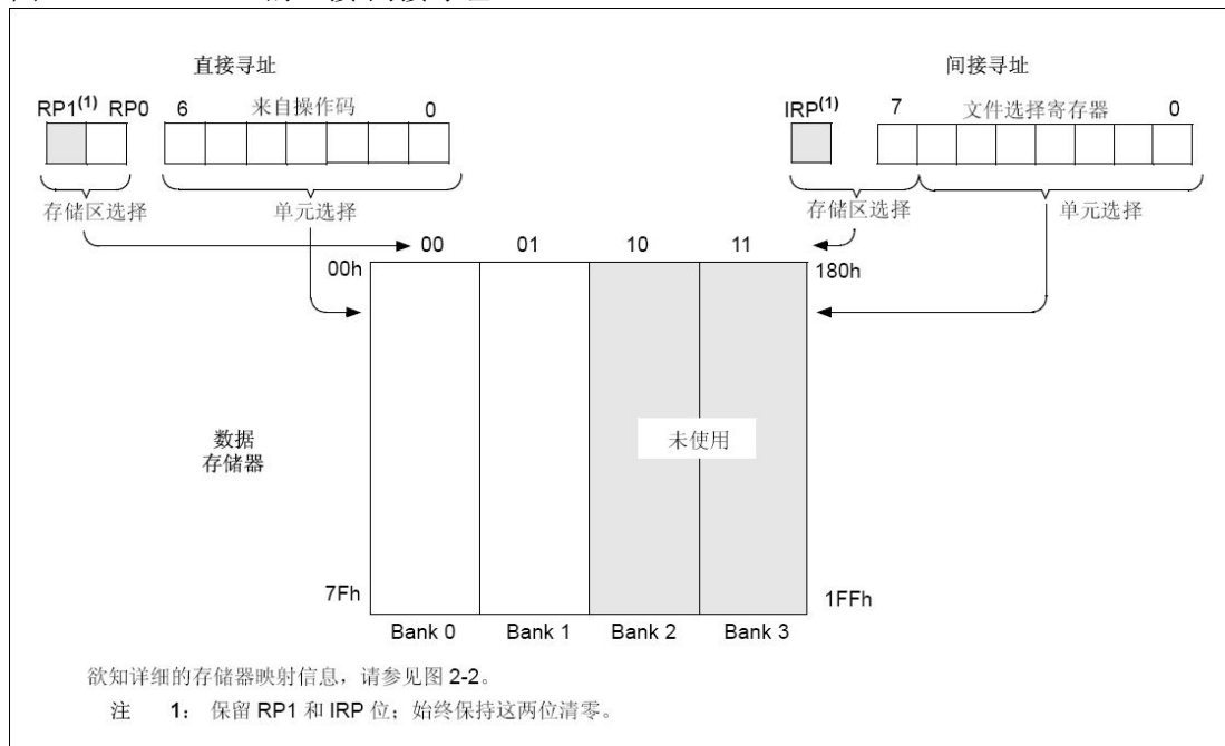
图 2-5: EN8F684 的直接/间接寻址
