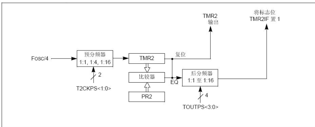
图 7-3: TIMER2 框图
