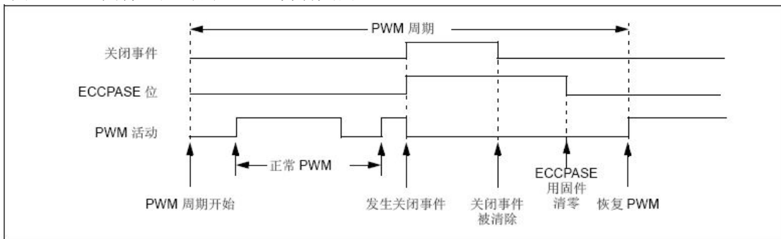
图 8-6-4: 固件重启时的 PWM 自动关闭 (PRSEN=0)
