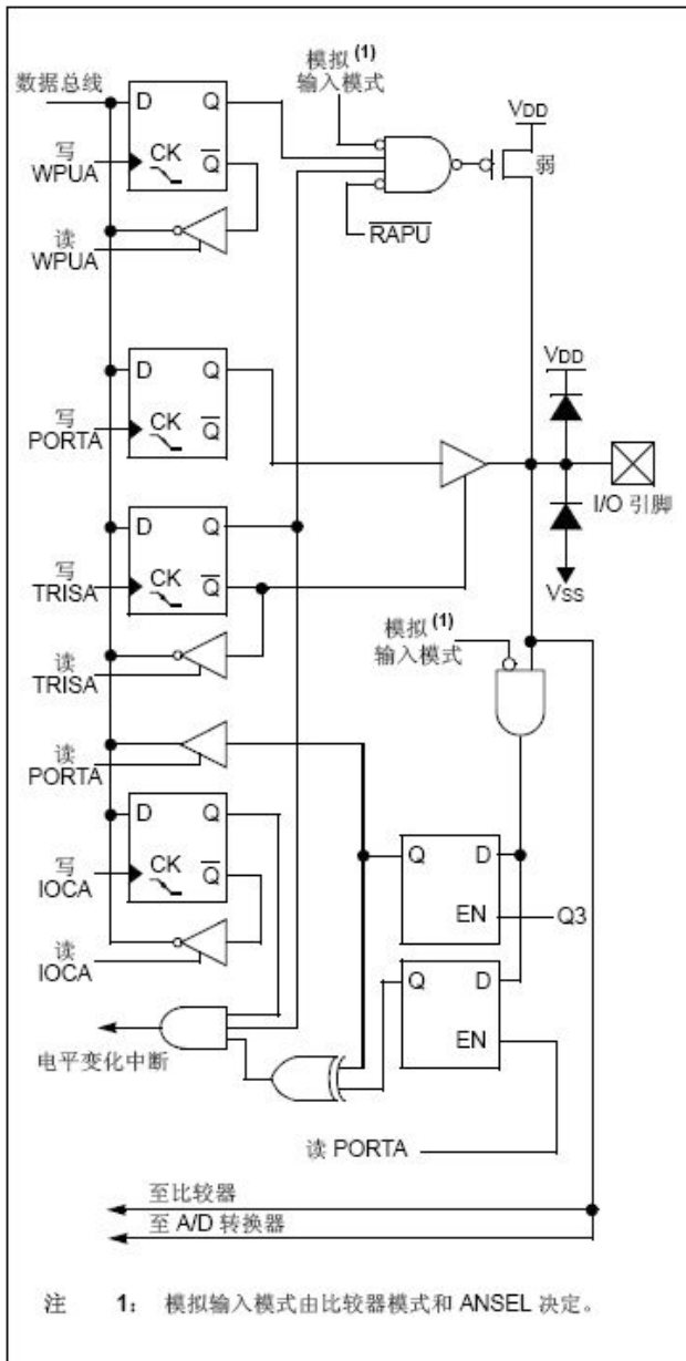
图 6-4-2: PA1 框图
