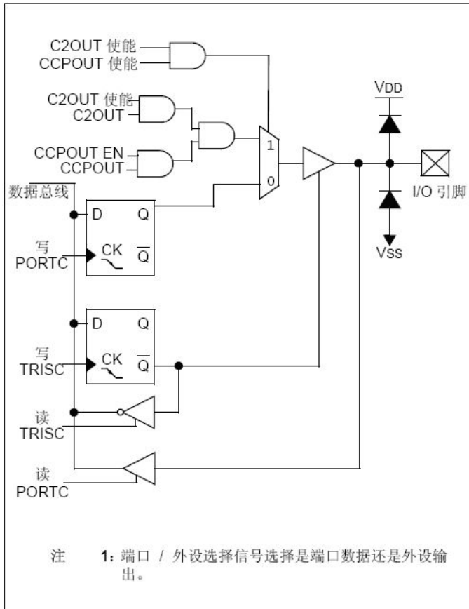
图 6-5-5: PC4 框图
