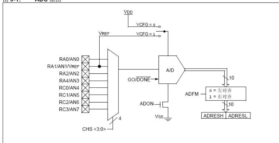
图 9-1: ADC 框图
