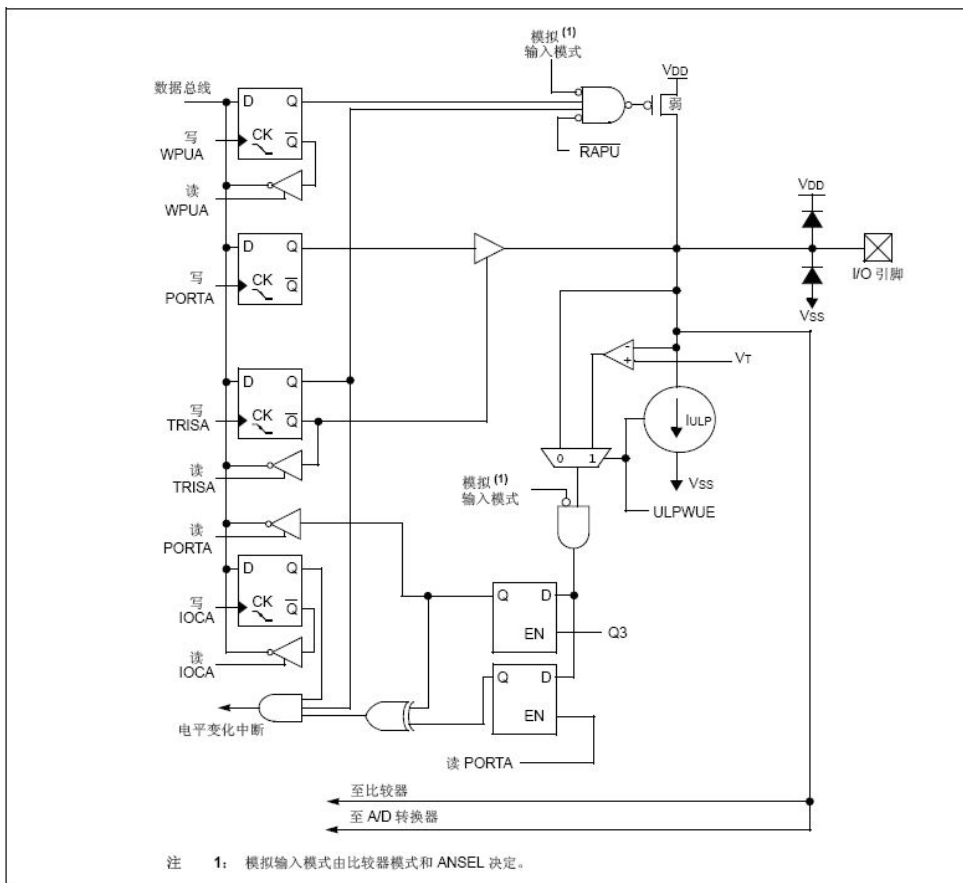
图 6-4-1: PA0 框图
