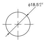
安装孔
