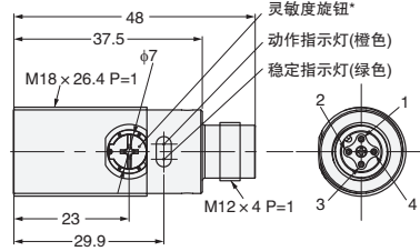
正视图
