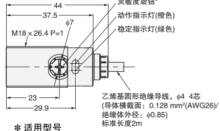
正视图
