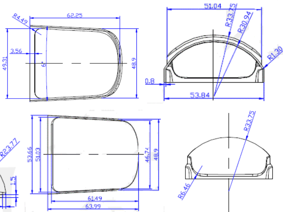
型号: Q10050, 焦距: 50mm, 角度: 120 度, 距离: 8m
