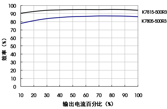
正输出效率Vs输出负载（标称输入）
