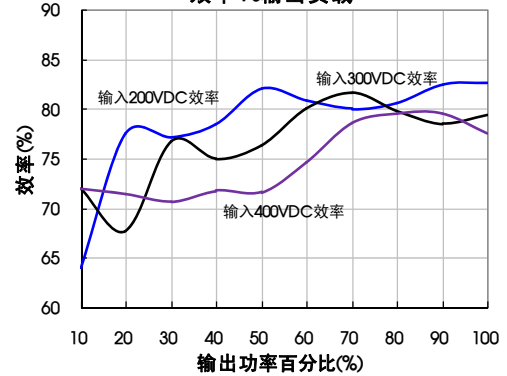
LS05-15B12SS DC 输入 效率Vs输出负载
