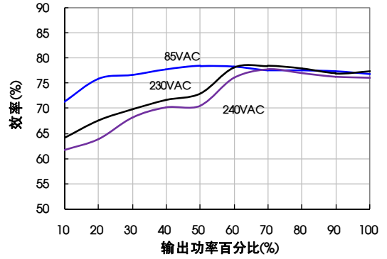
LS05-15B12SS AC 输入 效率Vs输出负载
