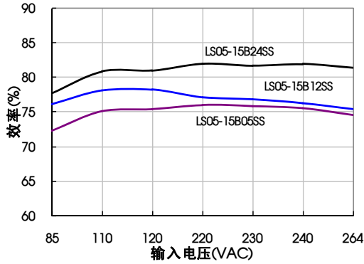
LS05-15BXXSS AC 输入 效率Vs输入电压(满载)
