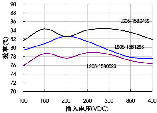
LS05-15BXXSS DC 输入 效率Vs输入电压(满载)
