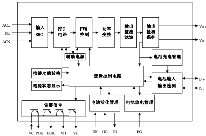
图1 电源内部原理图
