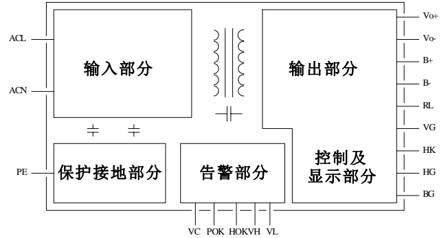
图2 电源内部隔离图
