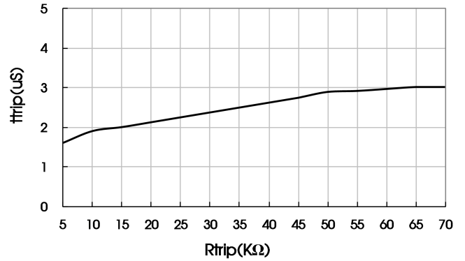
故障检测抑制时间与 R trip 关系的参考曲线
